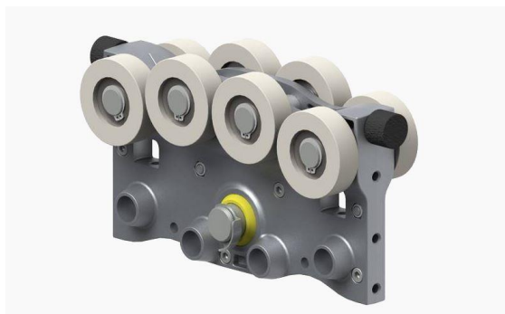
Závěsný vozík mostu jednoduchý.
